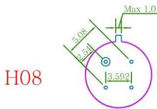
BOT VIEW
