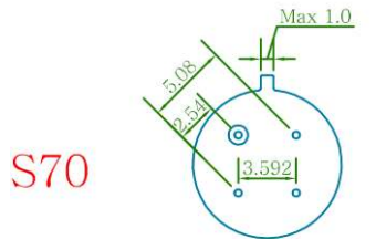
BOT VIEW
